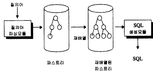
(그림 16) IDQL을 SQL로 변환하는 과정
