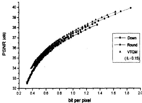
(그림 6) 양자화 방법에 따른 비트율과 PSNR (Lena 영상)
