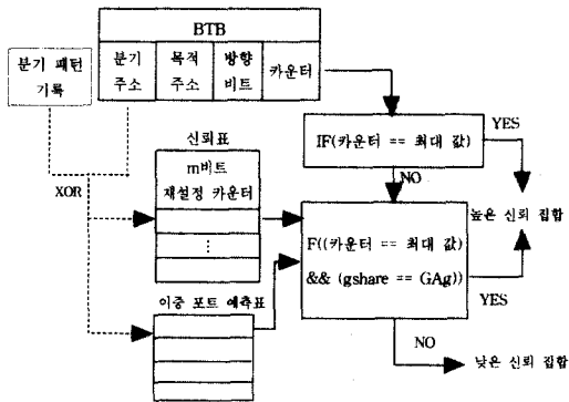
(그림 4) 통합 신뢰 메커니즘의 운영
