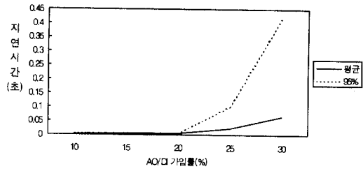
(그림 4) AO/DI 가입율에 따른 데이터 패킷 전송 지연시간
