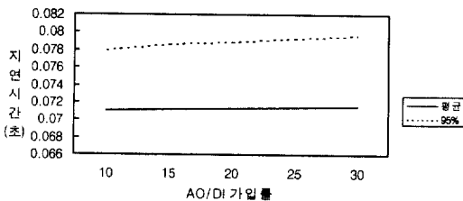
(그림 2) AO/DI 가입율에 따른 Q.931 호설정 지연시간
