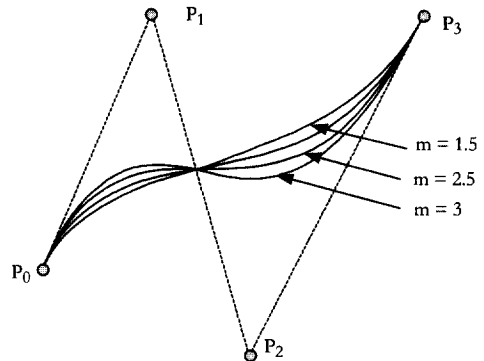
(Fig. 2) Variation of the Parameter m
