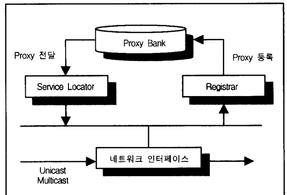
(그림 4) Lookup 모듈
