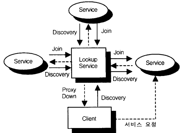
(그림 12) Jini Technology
