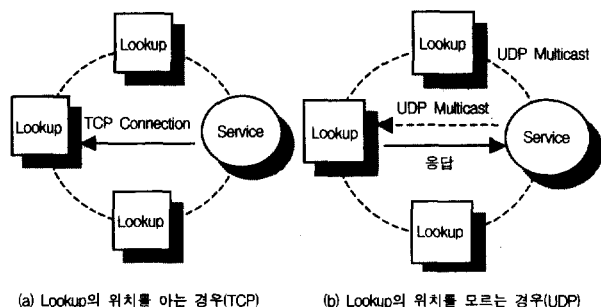
(그림 5) Service의 Lookup위치 파악
