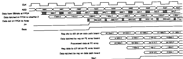
(그림 14) SRAM의 데이터 처리를 위한 타이밍도
