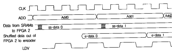
(b) 버퍼 2로부터 화면으로 전송되는 데이터 타이밍도
