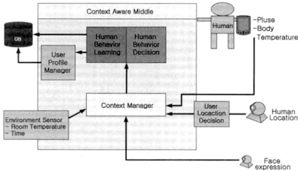
(그림 1) 상황인식 미들웨어 구성도
