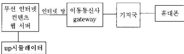
(그림 2) 정보 전달 시스템의 구조
