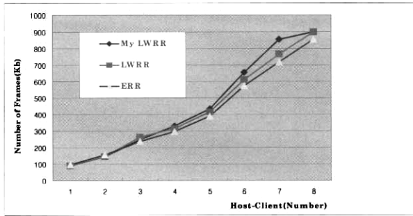
(그림 3) ERR/LWRR/My LWRR 패킷 데이터
