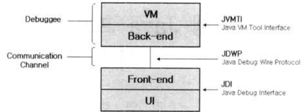
(그림 1) JPDA 구조도
