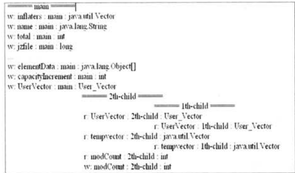
(그림 3) TFM으로 간단한 java 프로그램 실행결과
