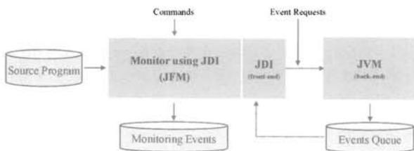
(그림 2) TFM (Transparent Filtering Monitor)의 수행환경
