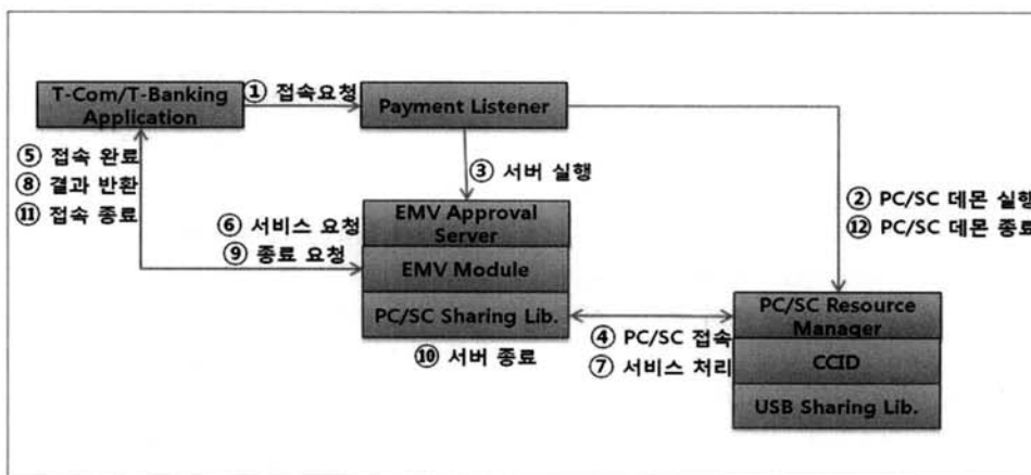
(그림 13) IC 신용카드 결제처리 모듈의 LifeCycle
