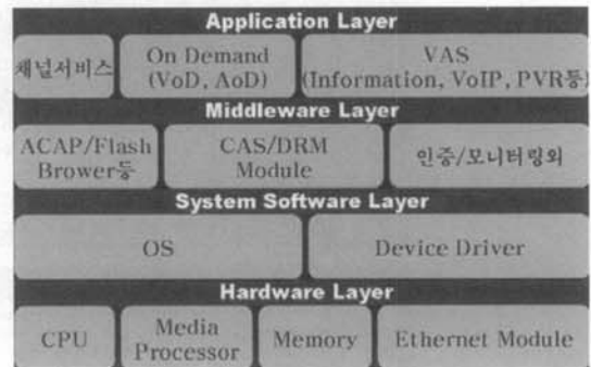
(그림 2) 셋탑박스 구성도
