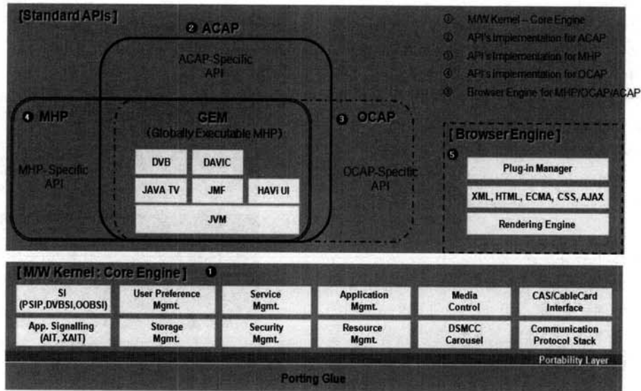
(그림 3) 미들웨어 구성도
