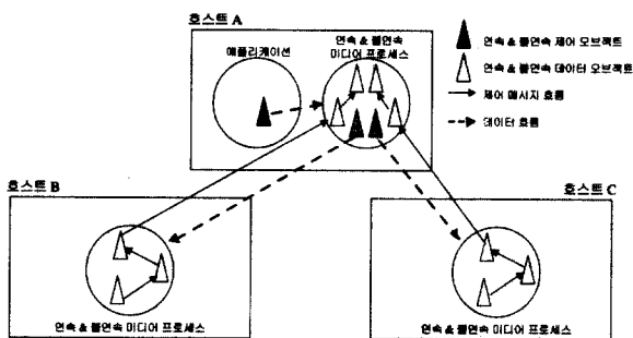
(그림 2) 확장-CMT로 작성한 응용의 구동 원리
