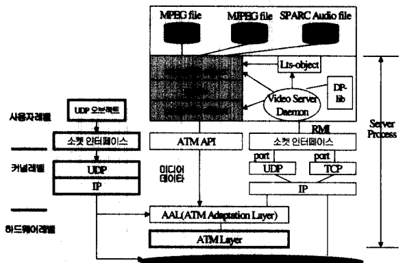
(그림 9) 확장-CMT를 사용한 미디어서버 구조
