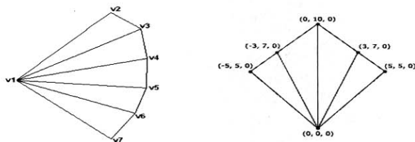
(그림 8) 삼각 팬(Triangle Fan)
