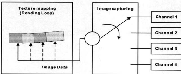
(그림 4) 영상 캡처 구조
