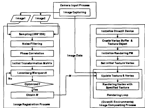
(그림 1) 고속 영상 모자이크 과정
