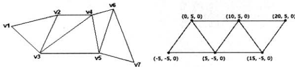
(그림 7) 삼각 스트립(Triangle Strip)
