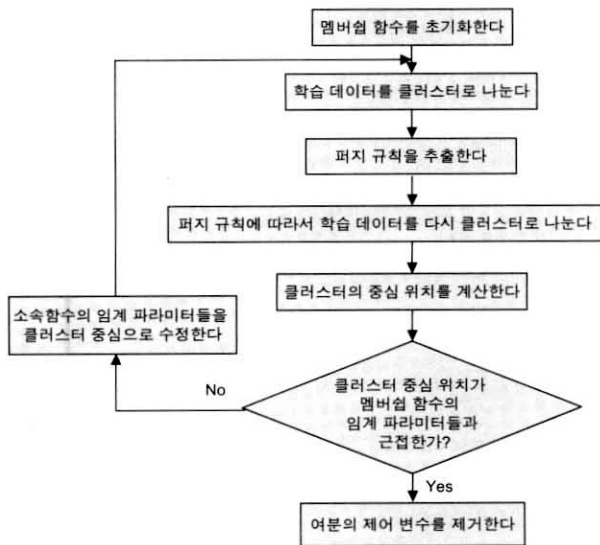
(그림 2) 퍼지 규칙 생성 알고리즘
