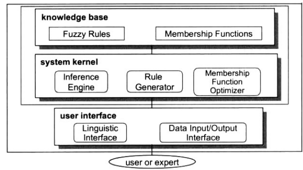
(그림 1) A-IDS-DAAP의 구조
