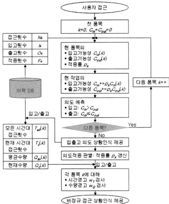
(그림 4) 로그기반 상황인식 알고리즘의 흐름도
