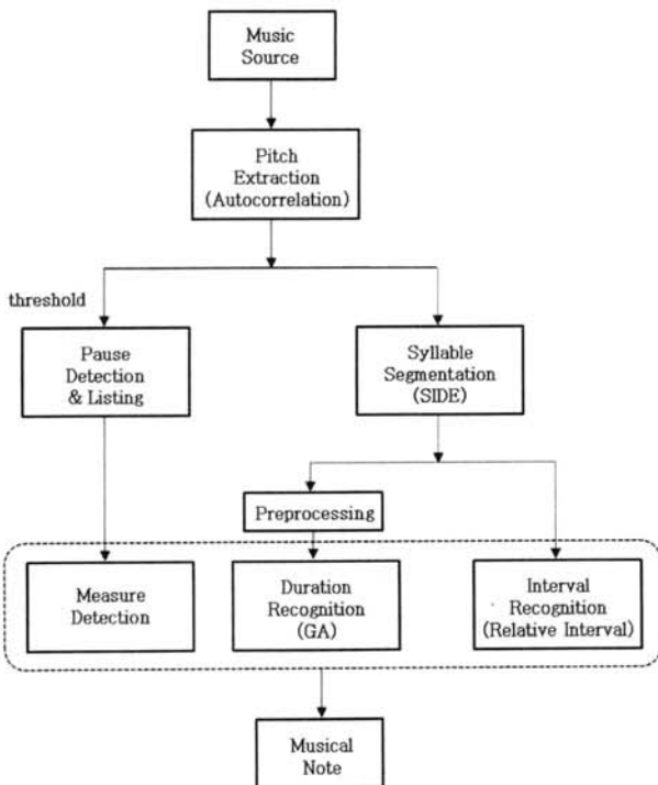
(그림 1) SIDE를 이용한 자동 음악 채보 시스템의 구조
