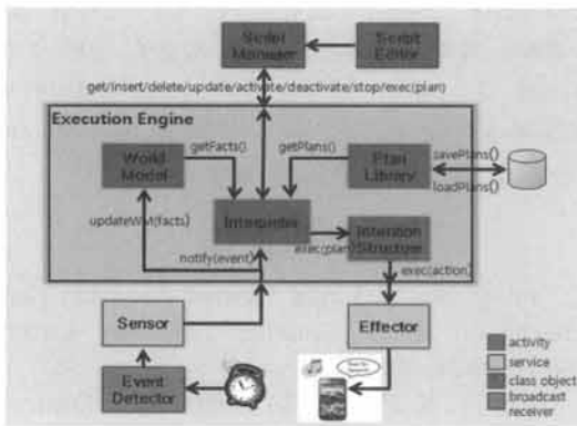
(그림 1) 스마트 스크립트 시스템의 구조
