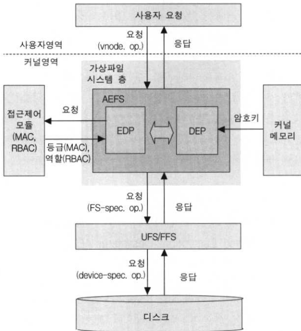
(그림 1) 접근제어 모듈이 적용된 AEFS 구조
