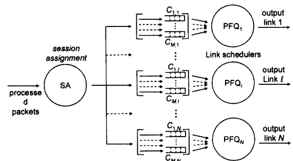
(b) SA-PFQ 모델
