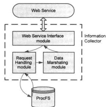
(그림 4) 정보 수집 데몬
