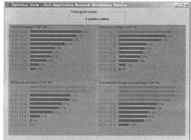
(그림 10) 통계정보 UI
