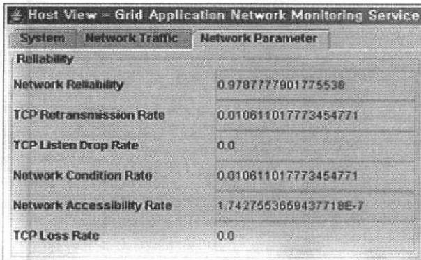
(그림 9) 네트워크 신뢰성 측정 UI
