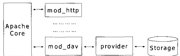
(그림 7) 아파치 mod_dav 모듈의 구조
