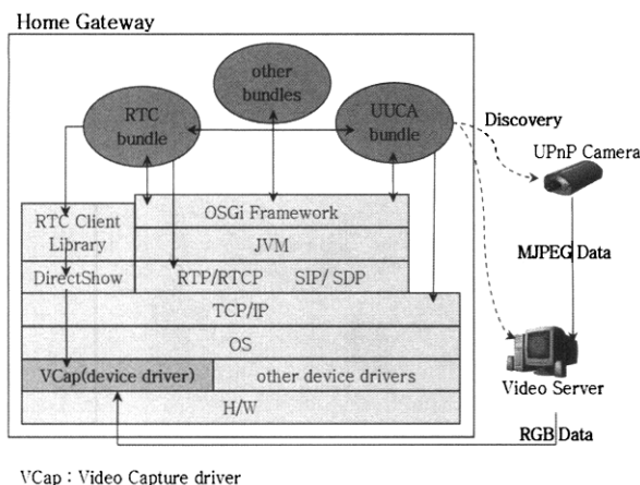
(그림 4) 홈 게이트웨이 소프트웨어 구조
