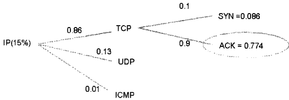
(그림 11) TCP ACK의 유용한 확률
