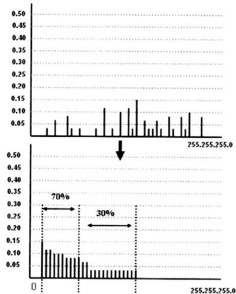
(그림 13) 트래픽 정보 DB에서 소스 IP 데이터 통계
