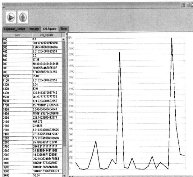
(그림 23) 카이제곱 값을 표시한 그래프
