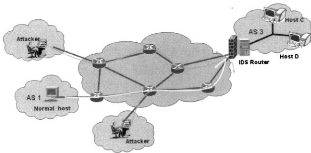
(그림 7) DDoS 대응시 정상호스트도 차단
