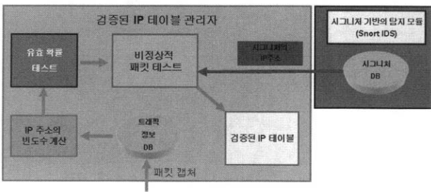
(그림 12) 검증된 IP 테이블 구조
