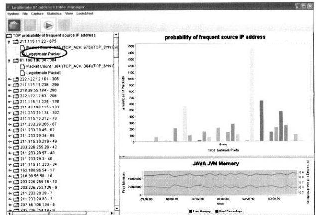
(그림 25) 검증된 IP 테이블 모듈
