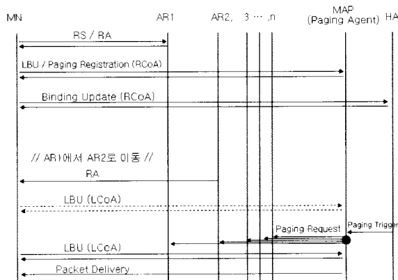
(그림 1) PHMIPv6에서 이동노드의 동작 및 페이징 메카니즘
