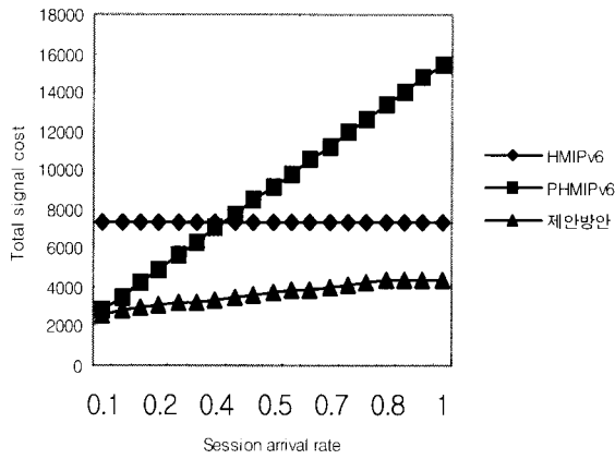
(그림 5) 세션 수신률에 따른 비용분석
