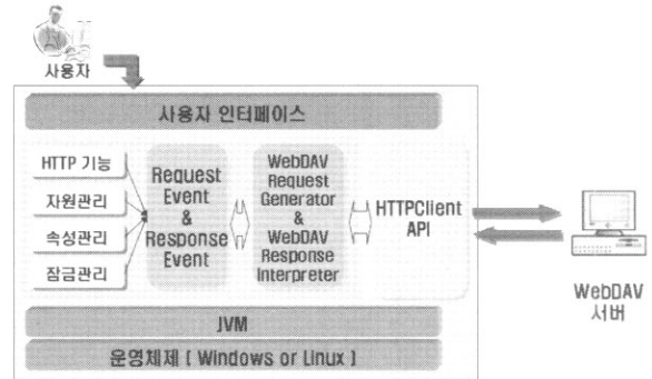
(그림 7) OpenDAVExplorer 클라이언트 구조
