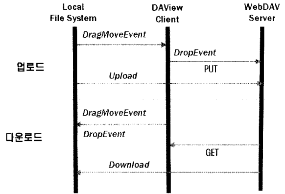
(그림 6) Drag & Drop 처리 과정
