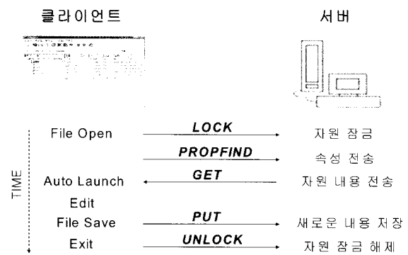
(그림 1) 웹데브 클라이언트의 프로토콜 요청 절차
