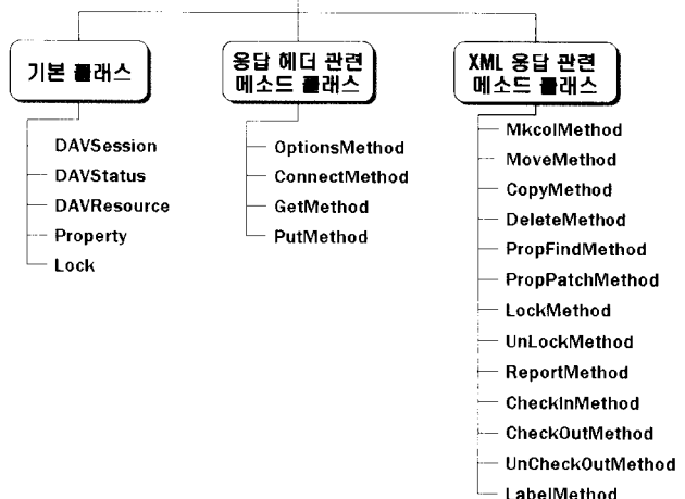
(그림 5) DAVon 라이브러리의 클래스들
