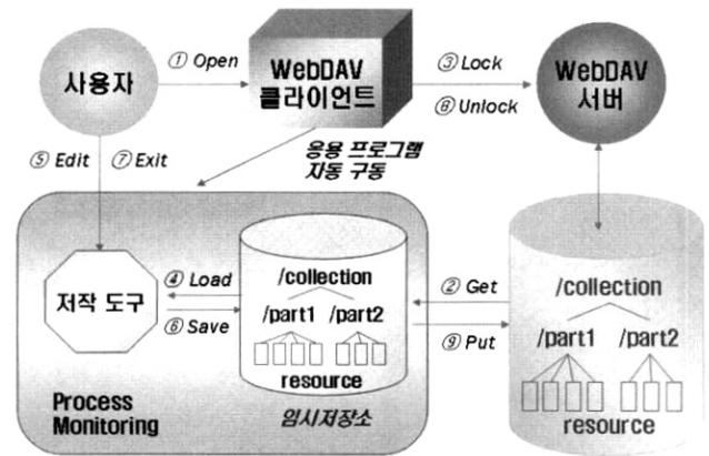
(그림 8) 클라이언트의 저작 처리 절차
