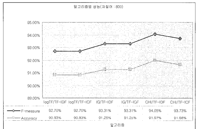
(그림 2) 알고리즘별 성능 (한글 자질어 800개)
