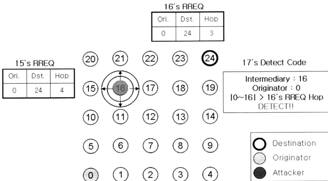
(그림 7) RREQ 메시지 변조 탐지
