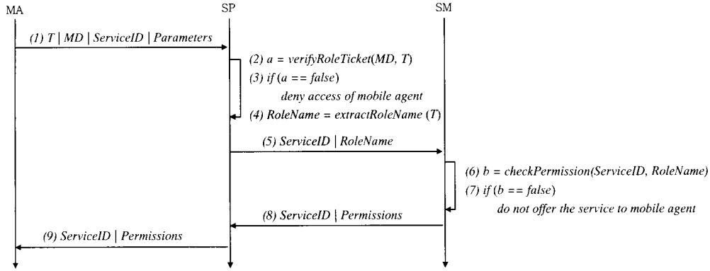
(그림 8) 플랫폼에서의 접근 제어 프로토콜
