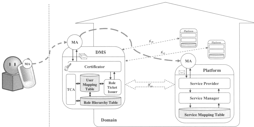
MA : Mobile Agent, DMS : Domain Management Server, TCA : Table Control Agent, K_m : Shared Key
