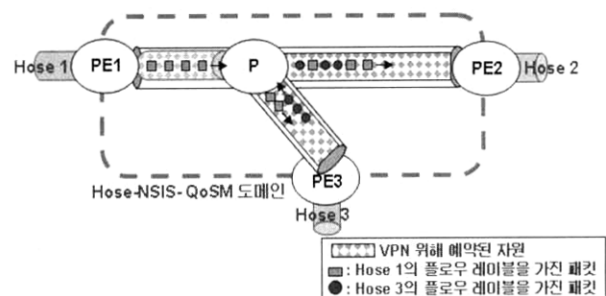
(그림 18) Hose 플로우 레이블과 VPN 별 데이터 전달
