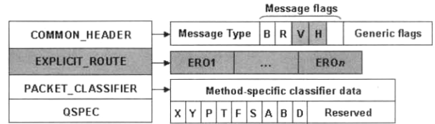
(그림 9) QUERY 메시지의 형태
