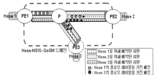
(그림 17) Hose 별 플로우 레이블과 Hose 별 데이터 전달
