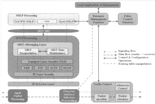
(그림 1) NSIS 시그널링의 프레임워크
