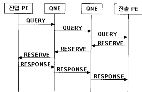
(그림 20) 수신자 시작 방법을 이용한 Hose-NSIS-QoSM에서의 시그널링 메시지
