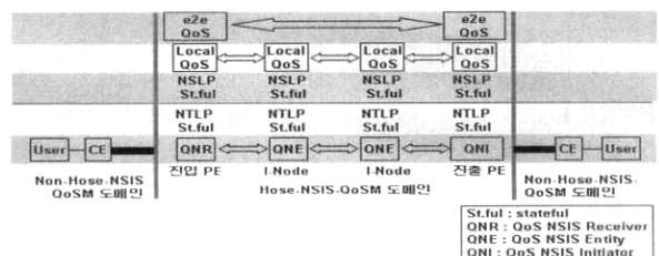
(그림 5) Hose-NSIS-QoSM에서의 상태 정보 프로세싱을 위한 프로토콜 모델
