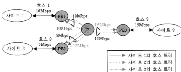
(그림 3) VPN-specific 상태 자원 준비에서의 자원할당
