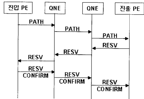
(그림 19) Hose-RSVP-TE-QoSM에서의 시그널링 메시지
