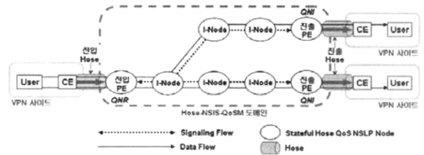
(그림 4) VPN과 Hose-NSIS-QoSM 도메인에서의 컴포넌트
