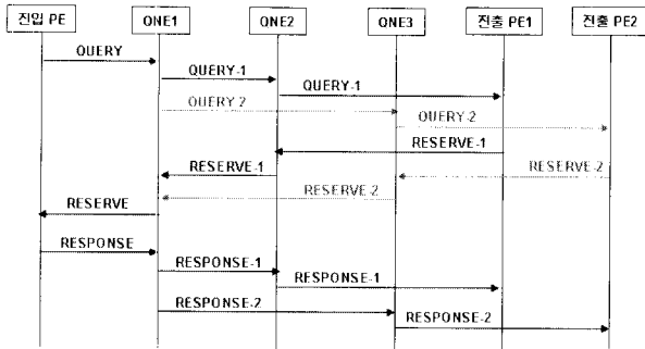
(그림 8) 시그널링 메시지 전달 과정
