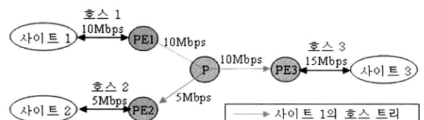
(그림 2) Hose-specific 상태 자원 준비에서 사이트 1의 Hose 트래를 위한 자원할당
