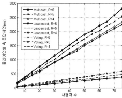
(그림 4) 서비스 요청-응답지연
