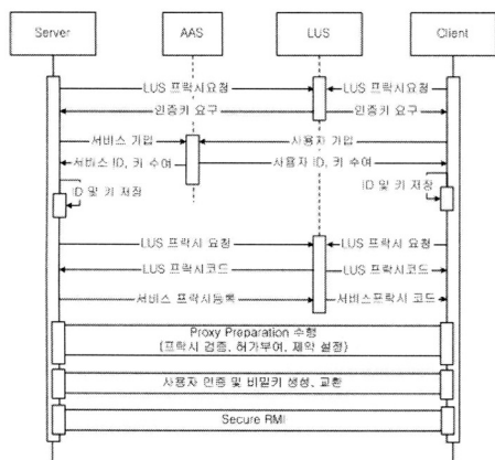
(그림 2) Jini 시스템 보안구조
