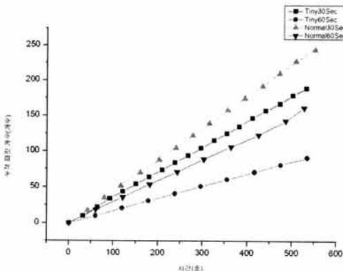
(그림 6) 데이터 요청 명령에 대한 패킷 수 (Fig. 6) Packet counts for data request
