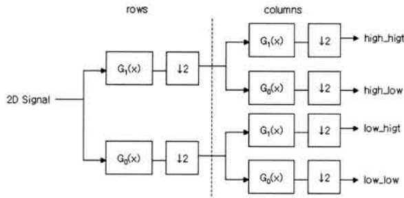
(그림 2) 분석 필터 뱅크
