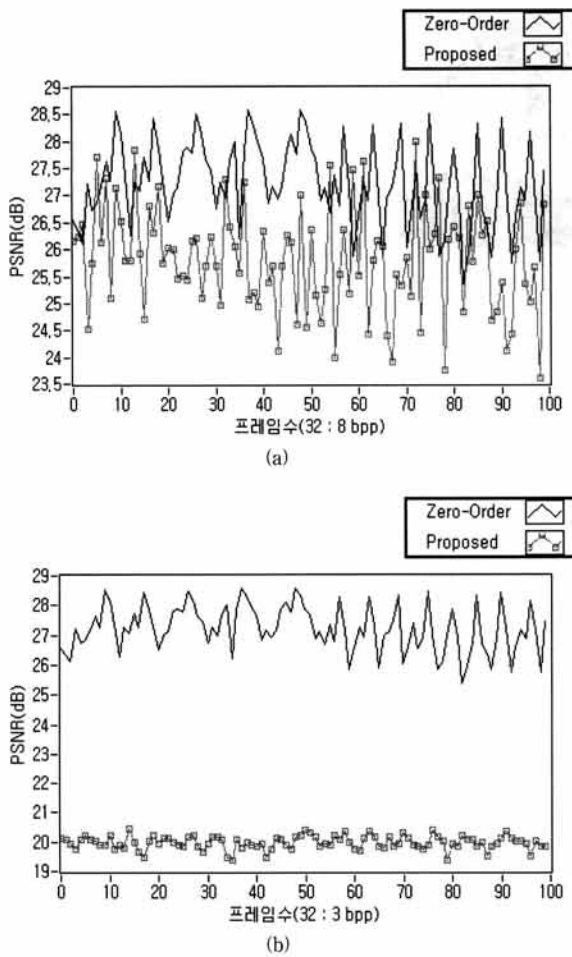
(그림 9) 프레임당 PSNR 성능 분석
