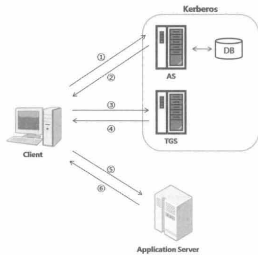
(그림 2) Kerberos의 인증 과정
