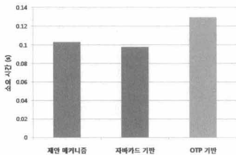
(그림 10) 메커니즘 간 인증 소요 시간 비교
