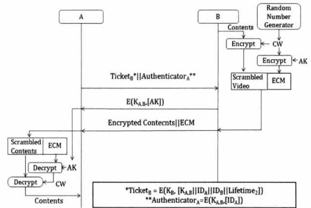
(그림 6) 서비스 요청
