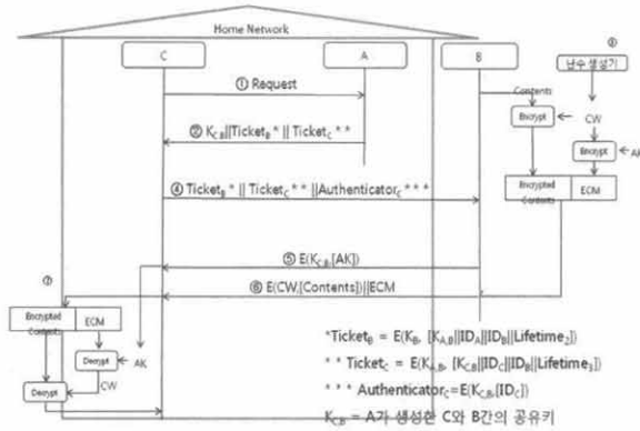
(그림 7) 기기 변경 및 맥내 티켓 재분배
