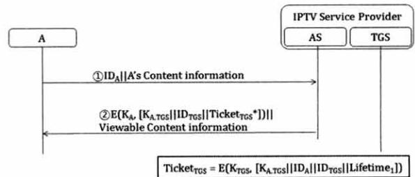
(그림 4) 콘텐츠 정보 전달 및 사용자 인증
