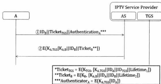
(그림 5) 티켓 발급 절차
