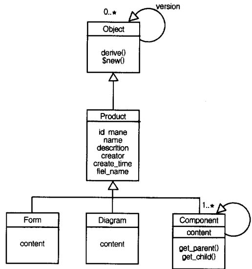
(그림 9) 객체 관계의 내부메타모델링의 UML 표현
