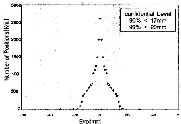
(그림 10) RTK-GPS의 고도에서의 위치 오차
