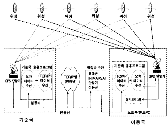
(그림 2) 전체 시스템 구성도
