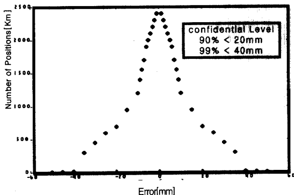
(그림 12) 동경에서의 오차율 비교
