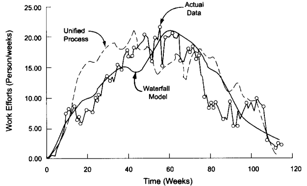
(그림 14) 개발인력 분포 추세 비교
