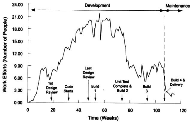
(그림 9) 소프트웨어 생명주기 투입인력 사례
