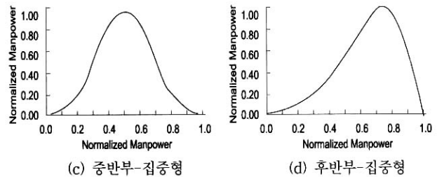
(그림 7) 가능한 소프트웨어 개발 인력 프로파일 형태
