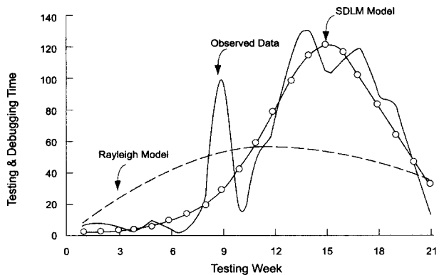
(그림 21) 시험과 디버깅 투입 인력의 실측치와 추정치
