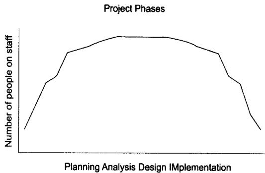
(그림 10) 전형적인 폭포수 프로세스의 인력 프로파일
