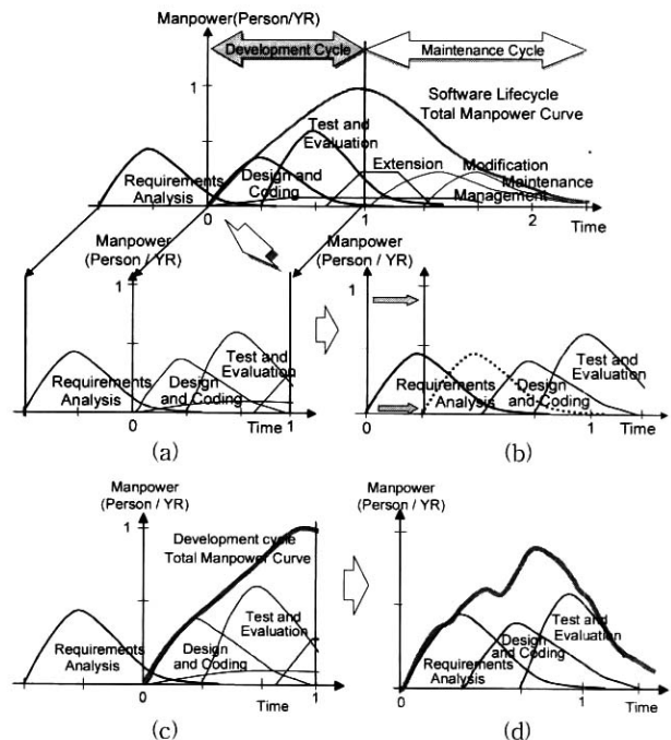
(그림 4) 폭포수 모델의 개발 인력 분포 유도
