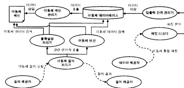
(d) 이동체 엔진의 입력력 흐름도
