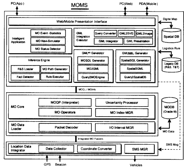
(그림 2) 이동체 관리 시스템 구조
