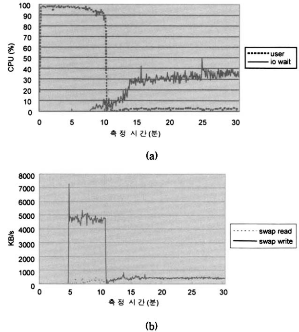
(그림 5) 메모리 위주 부하 생성 방식의 실험 결과
