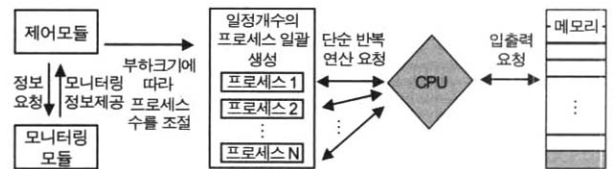
(그림 4) CPU 위주 부하
