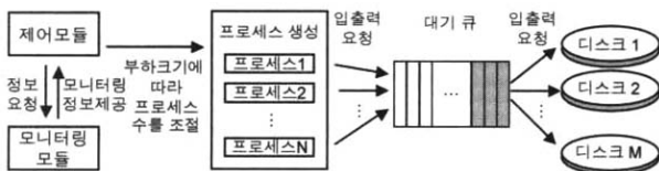
(그림 3) 입출력 위주 부하
