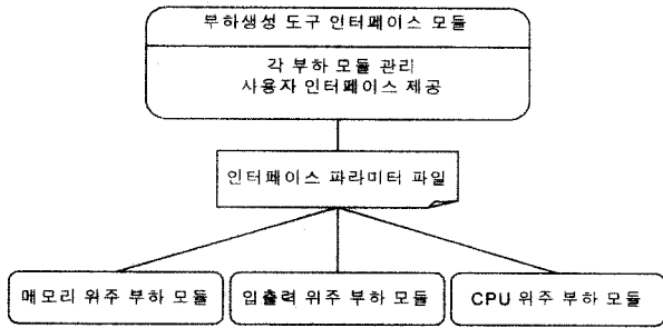
(그림 1) 부하 생성 도구의 모듈 구성
