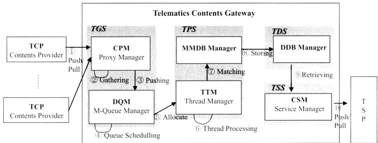
(그림 12) 텔레매틱스 콘텐츠 게이트웨이(TCG) 서브시스템 구성
