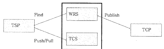
(그림 3) 텔레매틱스 콘텐츠 공개를 위한 웹 레지스트리 서비스 구조
