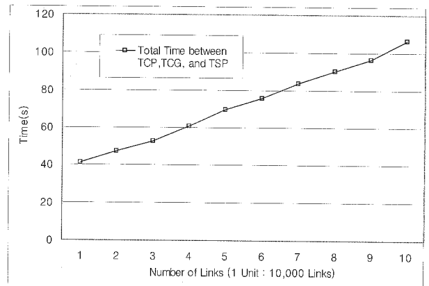
(그림 17) TCG의 성능 평가 : 링크수에 따른 소요시간
