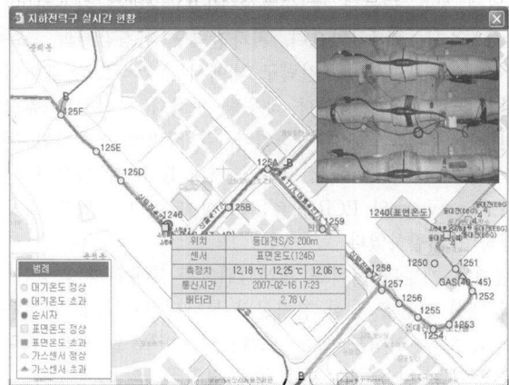
(그림 19) 지하전력구 모니터링 화면
