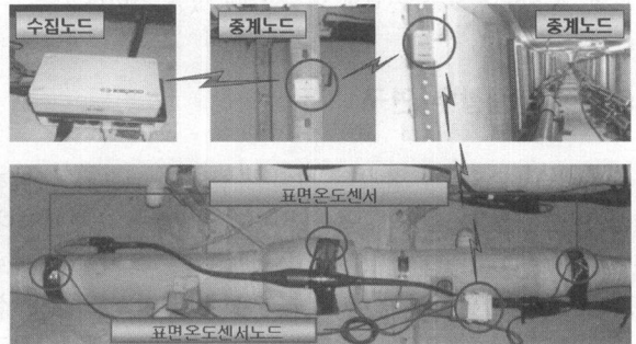
(그림 18) 전력구 및 접속함의 센서노드 설치 모습
