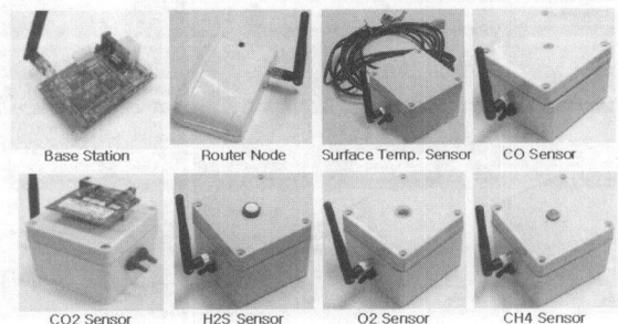
(그림 11) 지하전력구 감시를 위해 개발된 센서노드들
