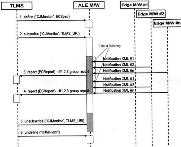
(그림 7) 미들웨어의 subscribe & publishing 방식
