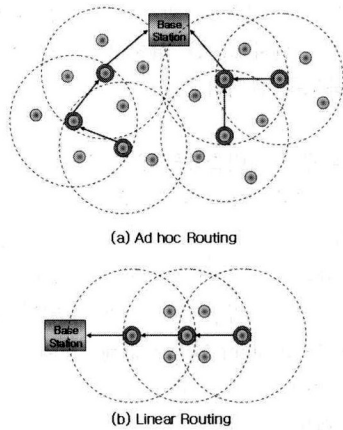
(그림 2) Ad hoc 라우팅과 직선형 라우팅
