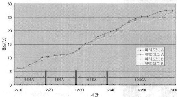
(그림 16) 파워도넛과 능동형 RFID 센서태그의 비교
