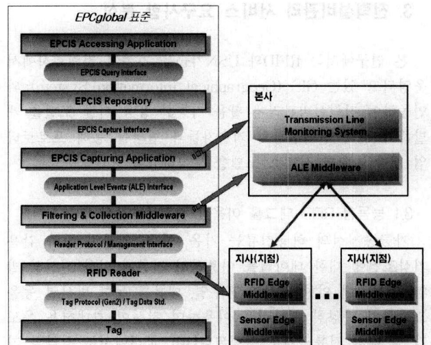
(그림 6) EPCnetwork를 응용한 프레임워크 적용 방안
