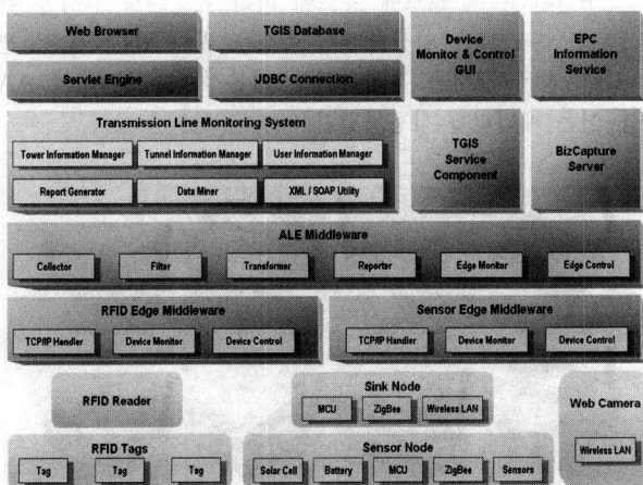
(그림 12) 전력설비관리서비스 프레임워크의 계층구조
