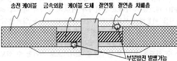
(그림 4) 케이블 접속함의 기본 구조
