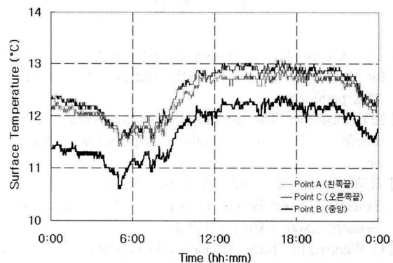
(그림 20) 접속함의 표면온도 변화그래프
