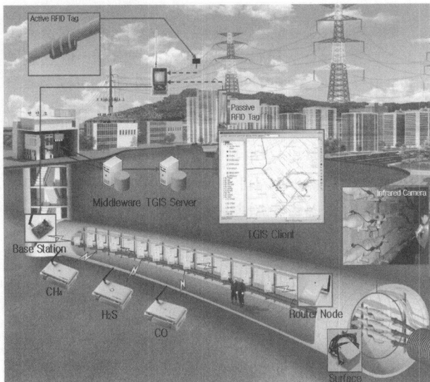
(그림 8) 전력설비관리 서비스 개념도
