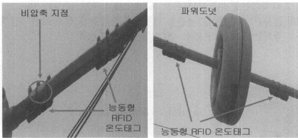
(a) 클램프 온도감시 (b) 송전선로 온도감시 (그림 15) 능동형RFID온도태그의 설치 모습
