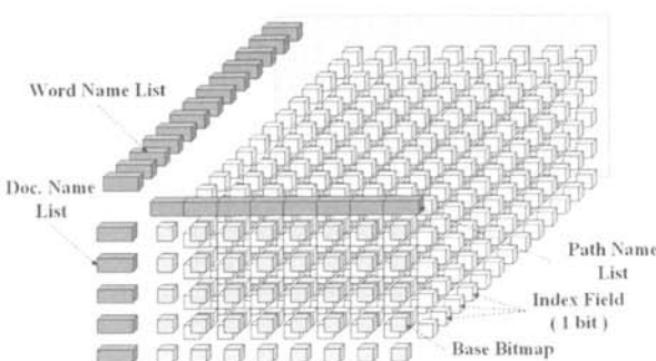
(그림 1) 3차원 비트맵인덱스(左)와 경로 비트맵인덱스(右)의 구조 비교
