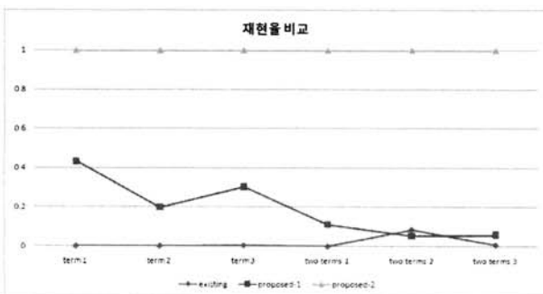
(그림 6) 재현율 비교 결과
