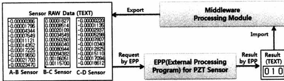
(그림 11) 구조물 건전성 감시 프로그램 연동된 PZT 데이터 처리 과정
