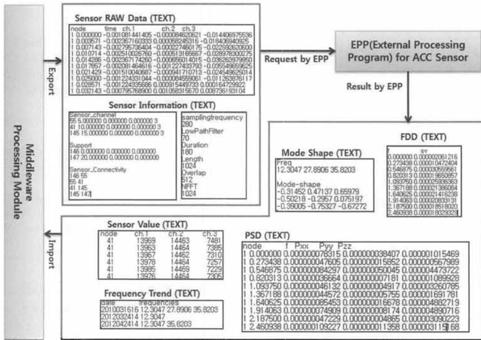
(그림 9) 구조물 건전성 감시 프로그램 연동된 ACC 데이터 처리 과정
