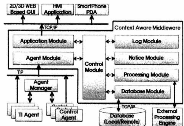
(그림 1) 상황 인식 시스템의 구성도
