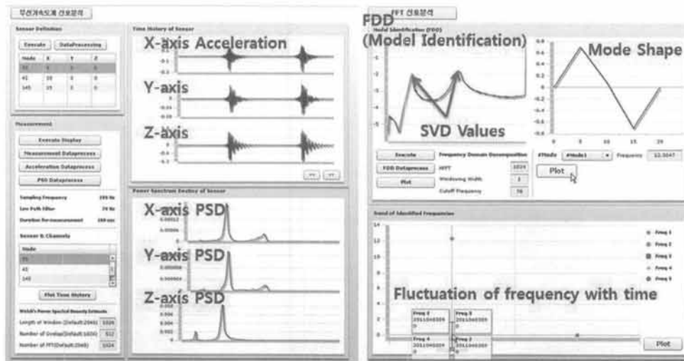
(그림 10) ACC 데이터 처리 결과의 웹 기반 UI
