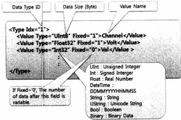
(그림 5) 상황 데이터 패킷의 XML 구조
