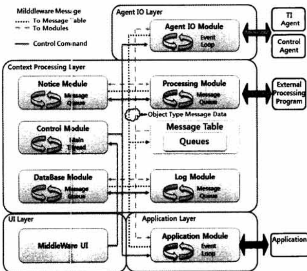
(그림 2) 상황 인식 미들웨어의 구조
