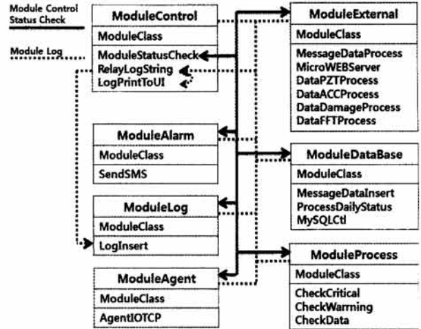
(그림 4) 모듈 클래스 구성과 제어 방법
