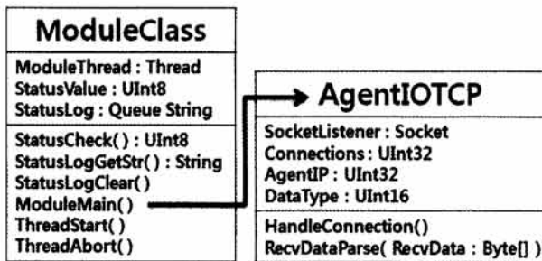
(그림 3) 에이전트 IO 모듈의 모듈 클래스
