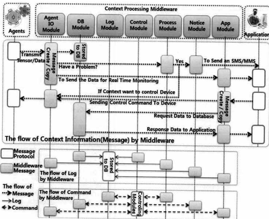
(그림 7) 미들웨어 메시지 처리과정
