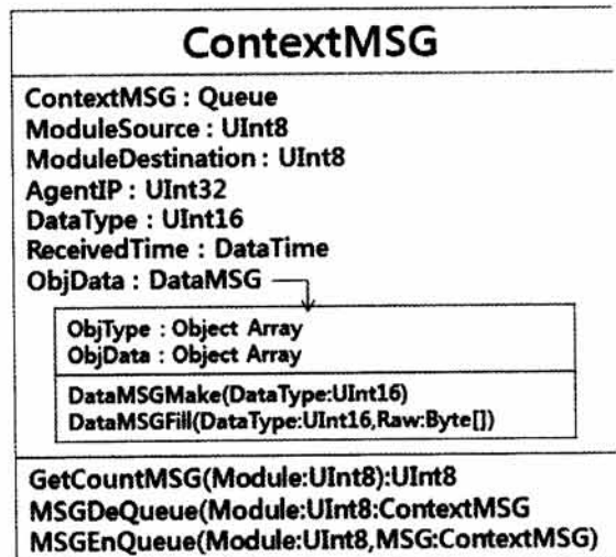
(그림 6) 미들웨어 메시지의 클래스
