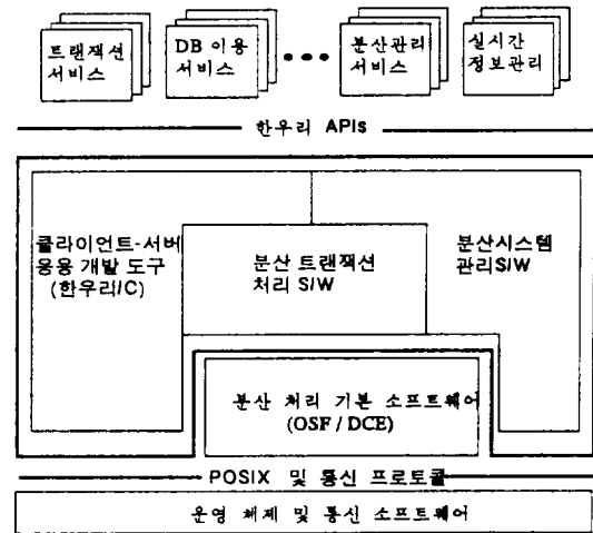
(그림 1) 한우리의 구성도 (Fig. 1) Structure of Hanuri
