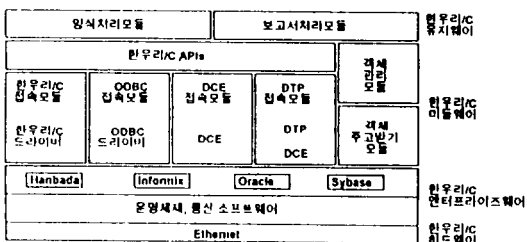
(그림 2) 한우리/C의 모듈 구성도 (Fig. 2) Block Diagram of Hanuri/C
