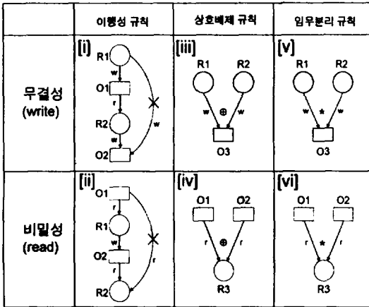
(그림 2) 보안 규칙의 분류 (Fig. 2) Classification of Security Constraints
