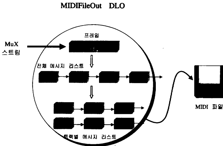
(그림 12) MIDI 파일 출력 DLO (Fig. 4) DLO for MIDI file output
