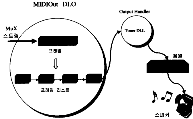
(그림 14) MIDI 출력 DLO (Fig. 6) DLO for MIDI output
