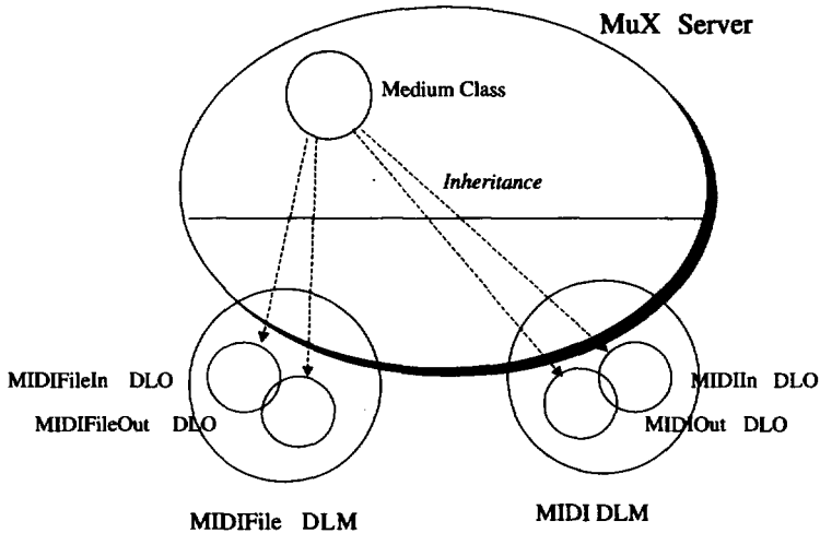
(그림 10) MIDI DLM의 구조 (Fig. 2) The architecture of MIDI DLM
